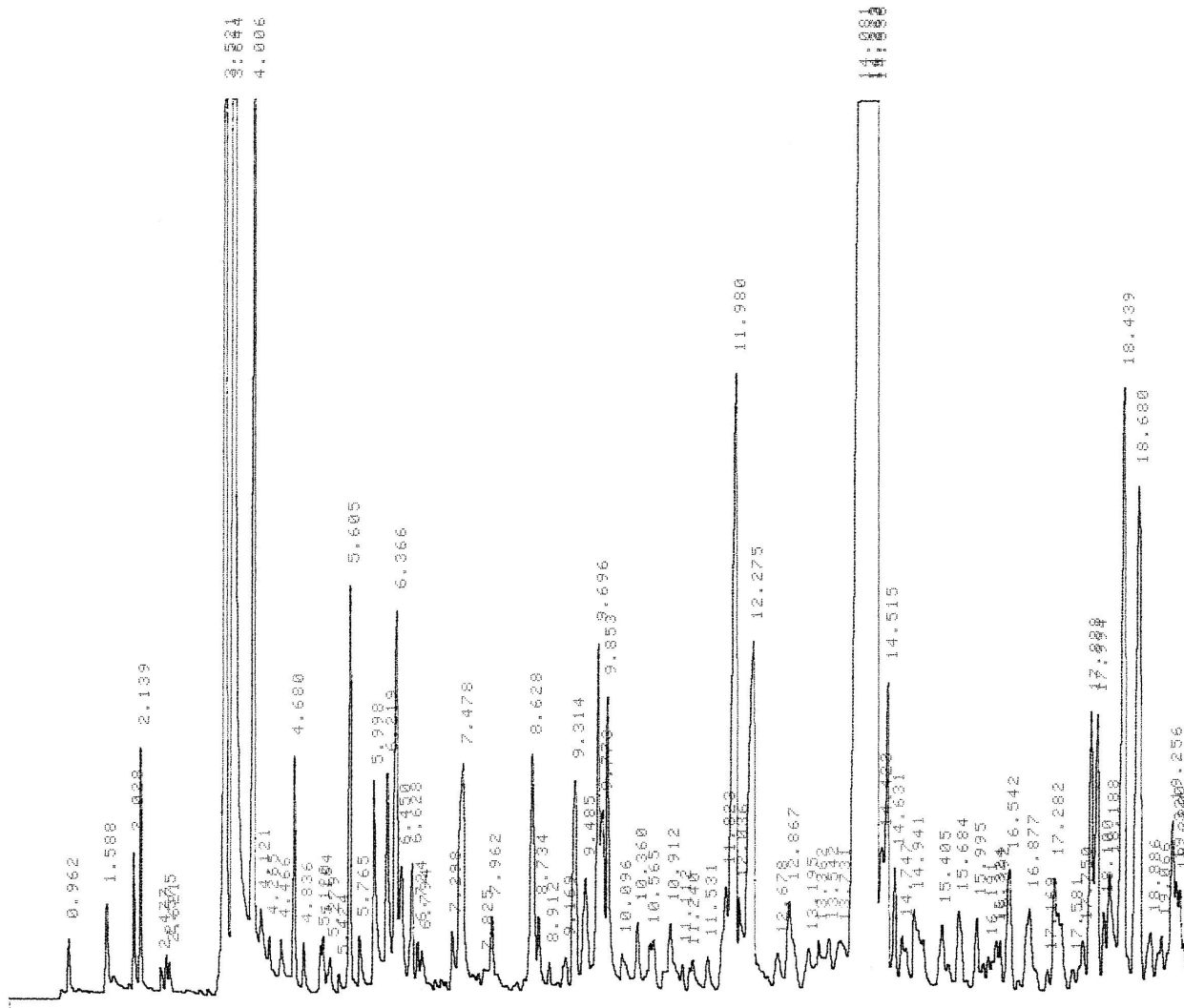
Figura 3 – Cromatograma de amostra do permeado.
