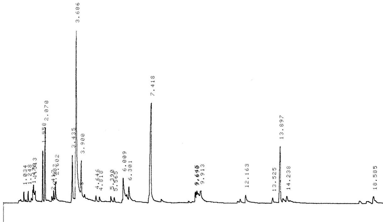
Figura 1 – Cromatograma de amostra da alimentação.
