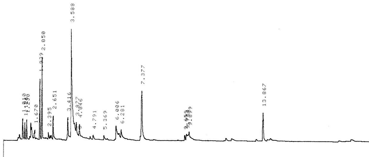
Figura 2 – Cromatograma de amostra do retido.
